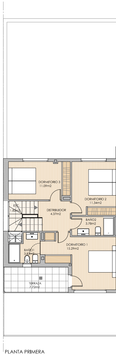
PLANTA PRIMERA
